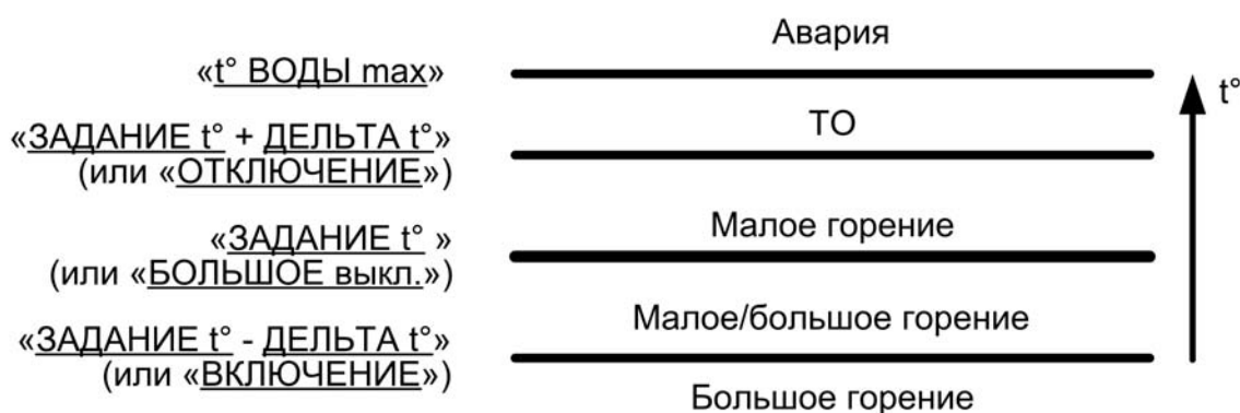
Рисунок 2 – Уставки температуры КУК-02
